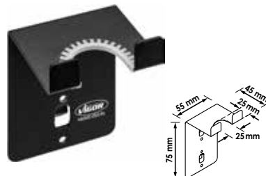
Drehmomentschlüssel-Halter · groß
