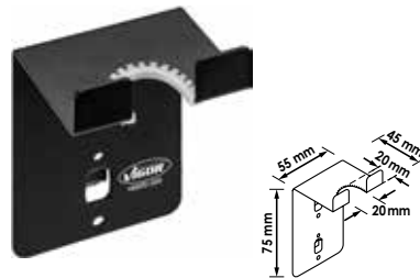
Drehmomentschlüssel-Halter
